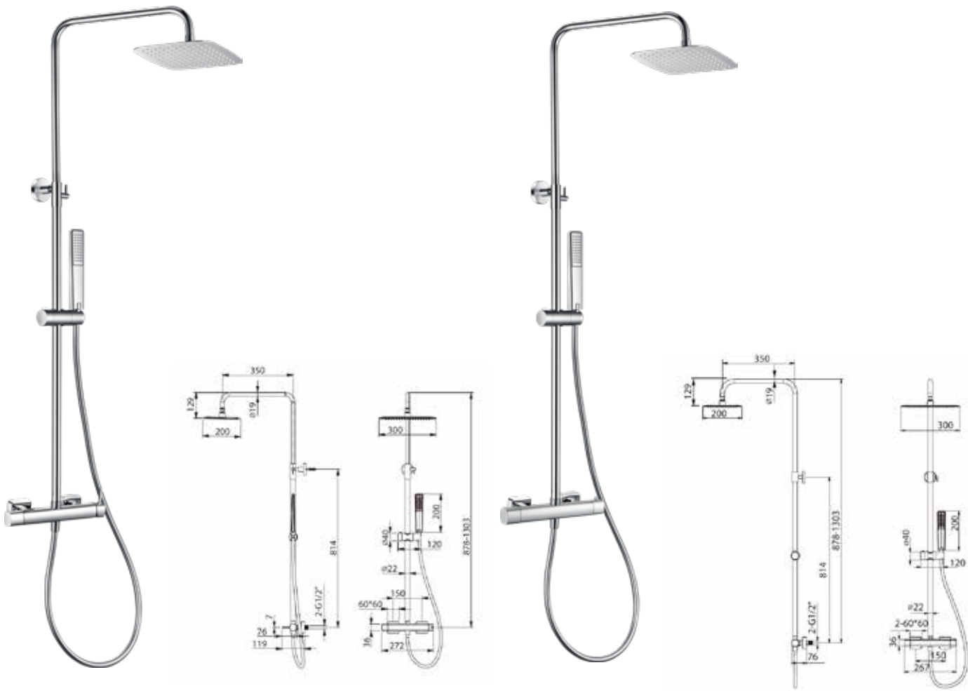
chrom DUÁLNI SPRCHOVÝ SYSTÉM TOSCANA
